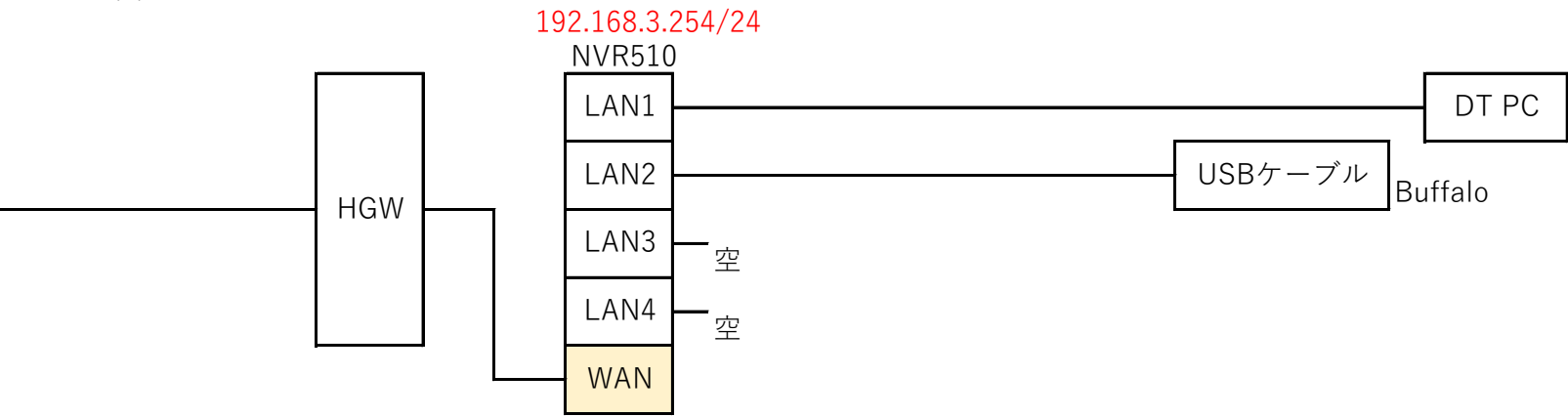
小牧構成図
